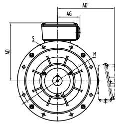
IM B5 (IM 3001) - V1 (IM 3011)
