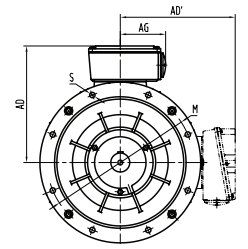
IM B5 (IM 3001) - V1 (IM 3011)
